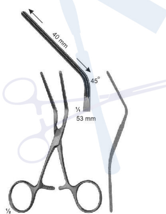
17-173 DE-BAKEY 45° winklig gebogen angled 45° 125 mm
